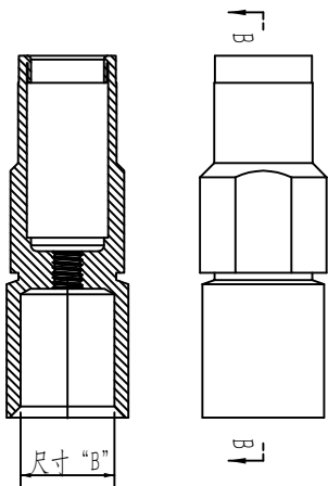
剖面视图 1 : 0.8
